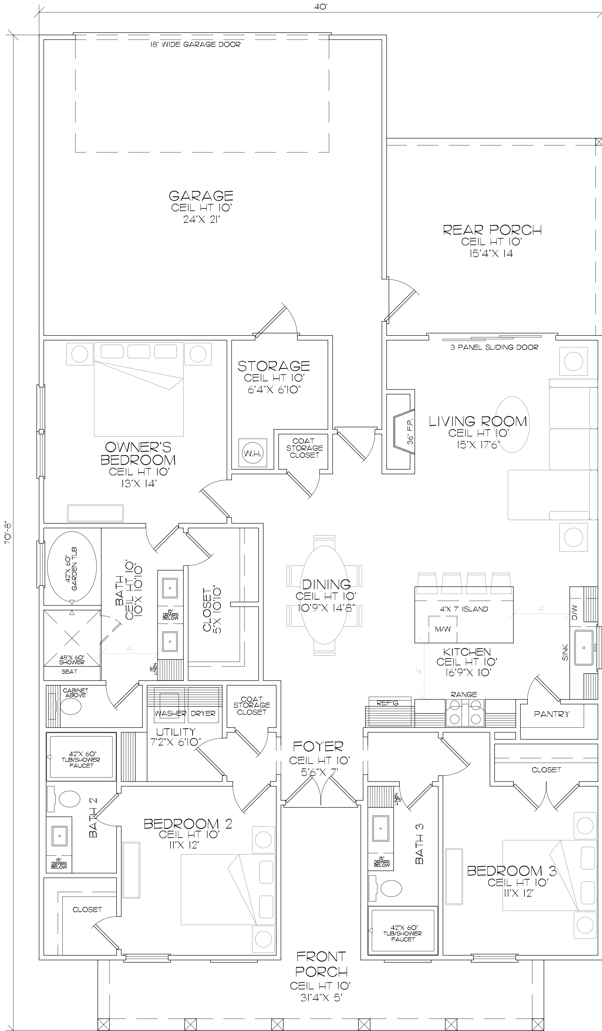
JAMESON_BENTLEY_CAMERON FLOOR PLAN SCALE: 1/4"= 1'-0"
